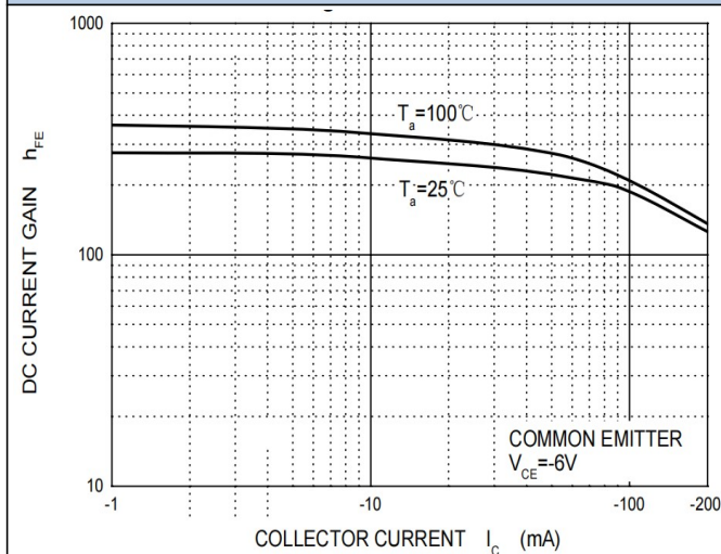
Fig.2 h_{FE} - I_C
