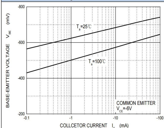
Fig.3 V_{BE} - I_C
