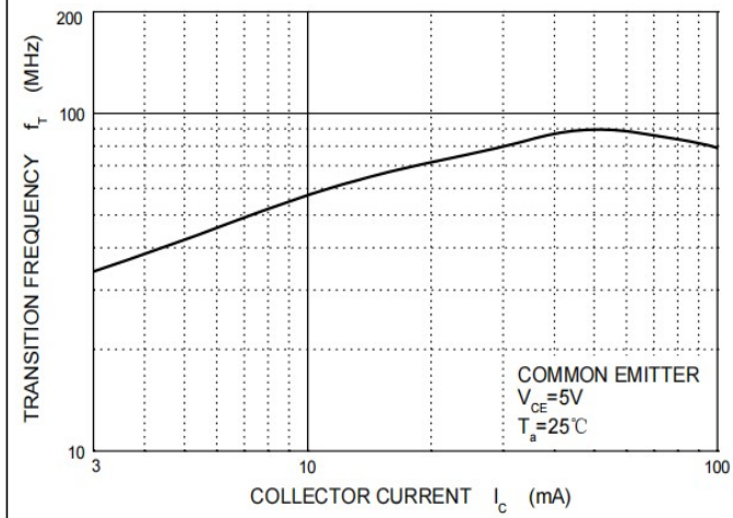
Fig.7 f_T - I_C
