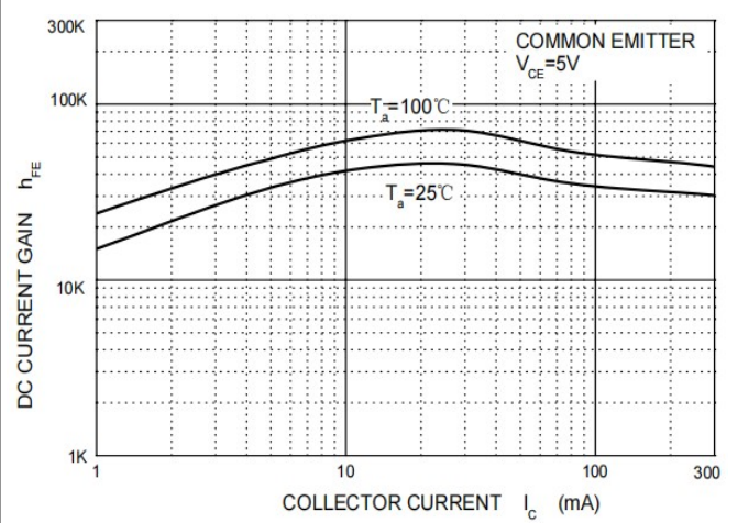
Fig.2 h_{FE} - I_C
