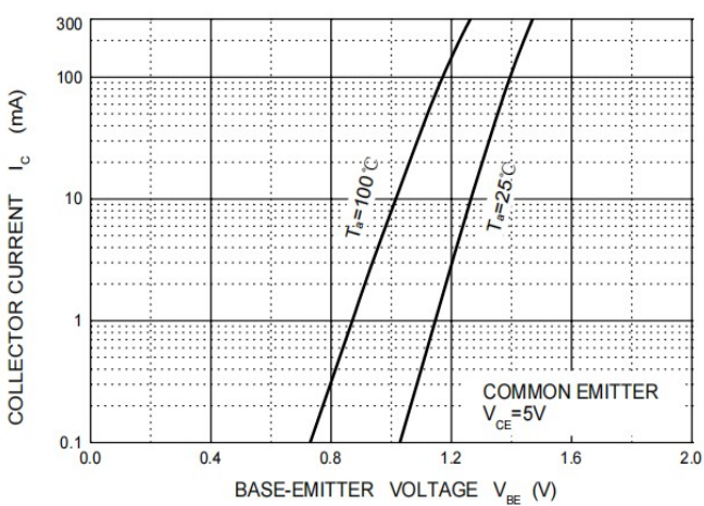
Fig.5 I_C - V_{BE}
