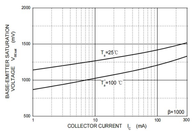
Fig.4 V_{BE(sat)} - I_C
