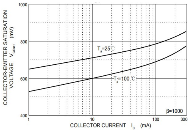
Fig.3 V_{CE(sat)} - I_C
