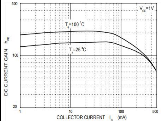
Fig.2 h_{FE} - I_C
