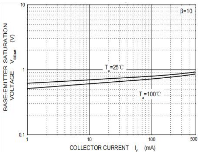
Fig.3 V_{BEsat} - I_C
