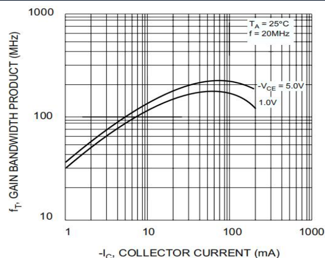
Fig.5 f_T - I_C
