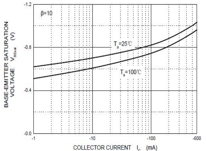
Fig.4 V_{BEsat} - I_C
