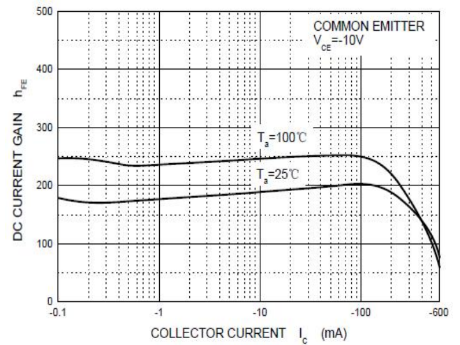
Fig.2 h_{FE} - I_C
