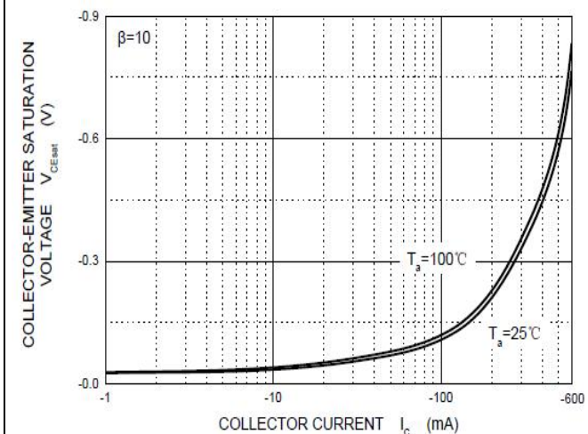
Fig.3 V_{CEsat} - I_C
