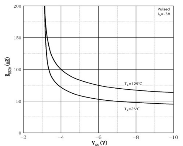
Fig.4 R_{DS(on)} - V_{GS}
