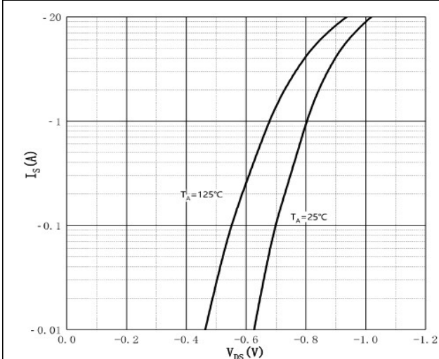
Fig.5 I_S - V_{SD}
