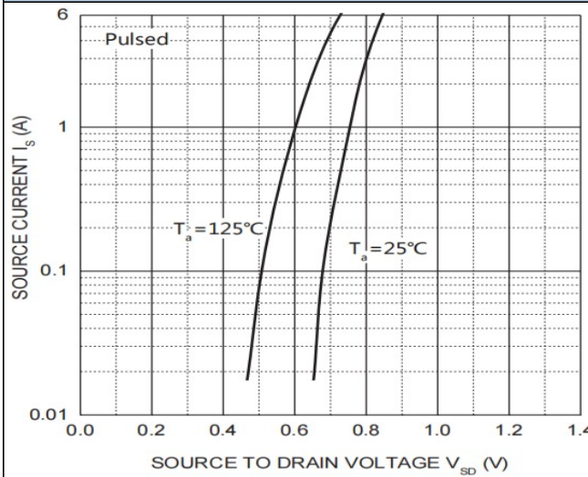
Fig.5 I_S - V_{SD}
