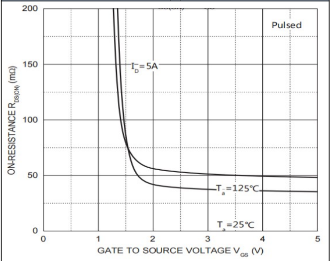
Fig.4 R_{DS(on)} - V_{GS}
