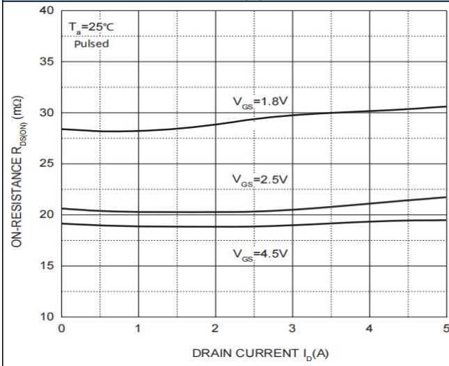
Fig.3 R_{DS(on)} - I_D
