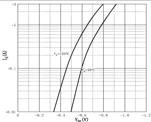
Fig.5 I_S vs. V_{DS}
