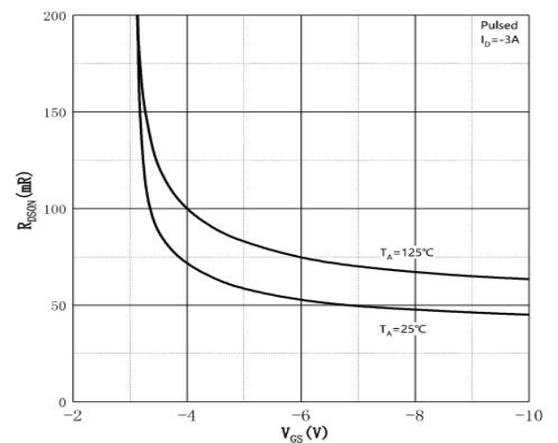
Fig.4 R_{DS(on)} - V_{GS}
