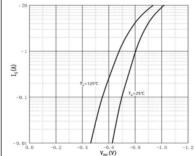
Fig.5 I_S - V_{SD}
