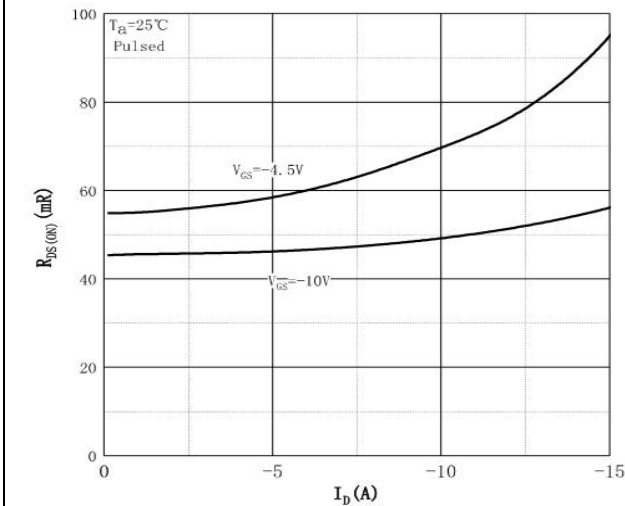
Fig.3 R_{DS(on)} - I_D
