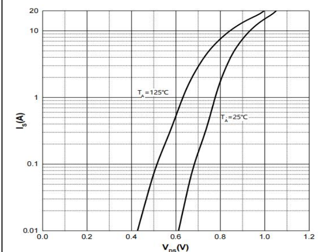
Fig.5 I_S - V_{SD}
